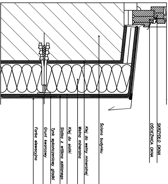
DETAL OBRÓBKI PARAPETU PRZEMKÓW PIONOWY
