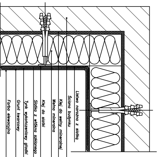
DETAL OCIEPLENIA NAROŻA WKŁĘSEGO PRZEMKÓW POZIOMY
