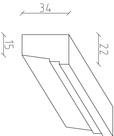
G1 -Gzyms nad parterem
