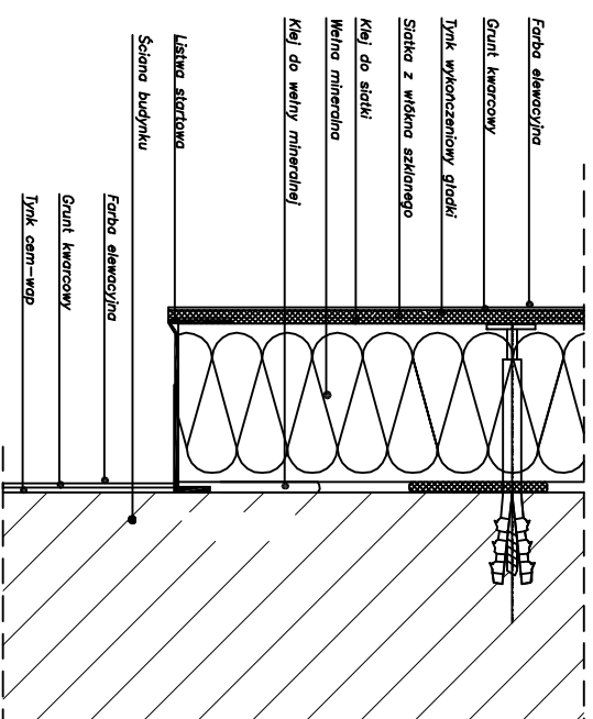
DETAL DOLNEJ KRAWĘDZI DOCIEPLENIA PRZEKRÓJ PIONOWY
