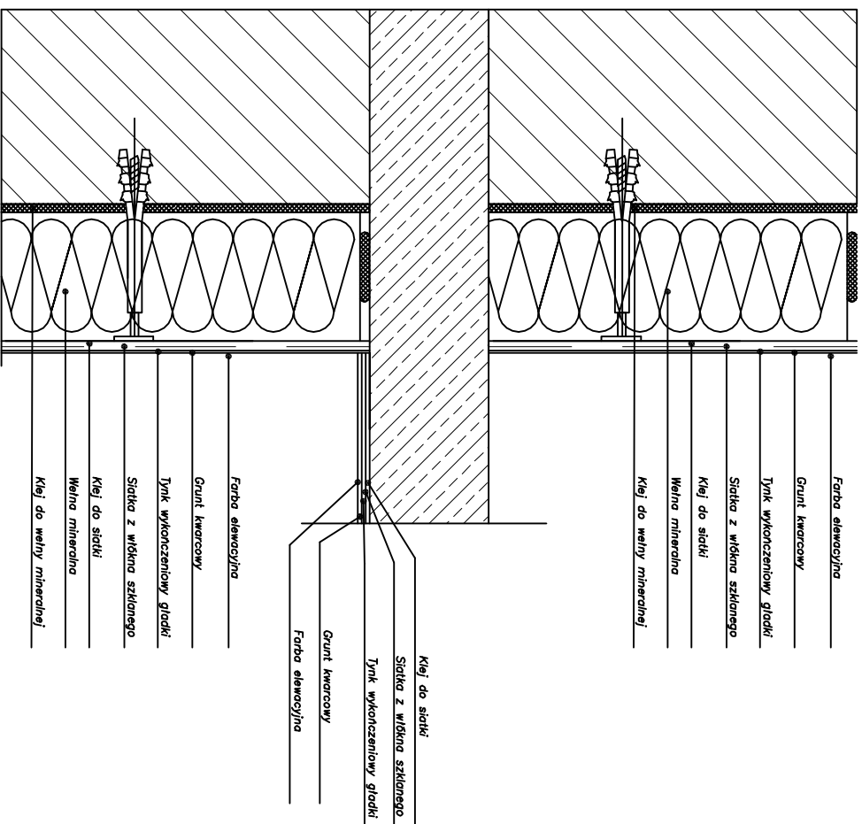
DETAL OCIEPLENIA ŚCIANY PRZY POŁĄCZENIU Z BALKONEM PRZEKRÓJ POZIOMY
