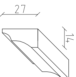
G2 Gzyms wieńczący
